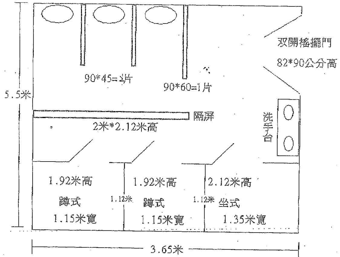
廁所隔間板示意圖
