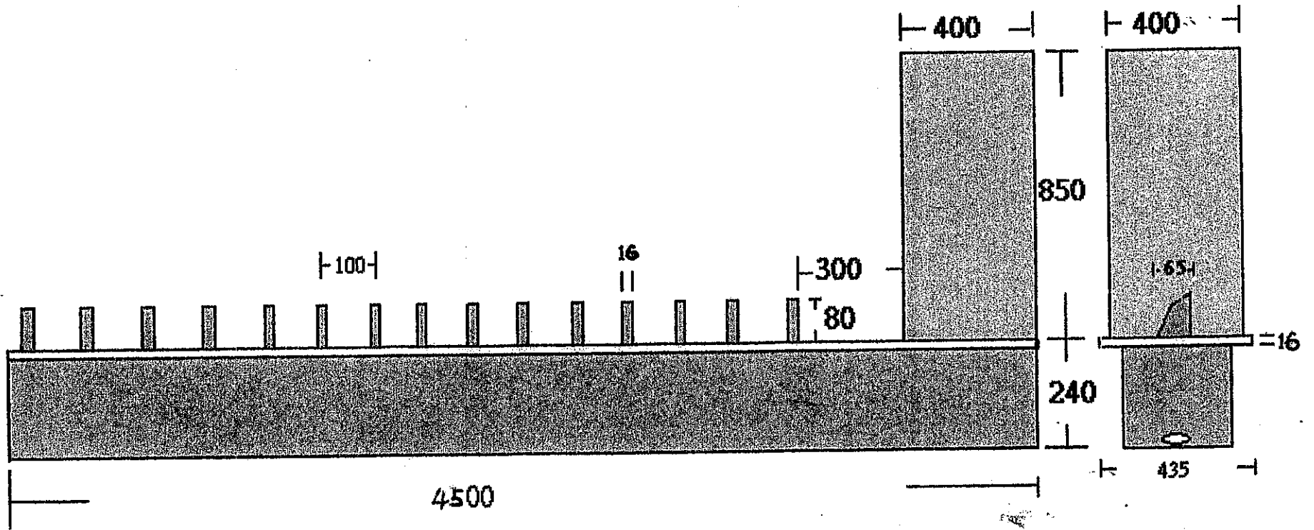
阻車柵詳圖 1
