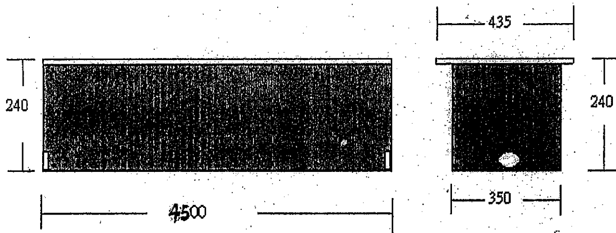
阻車柵詳圖 2
