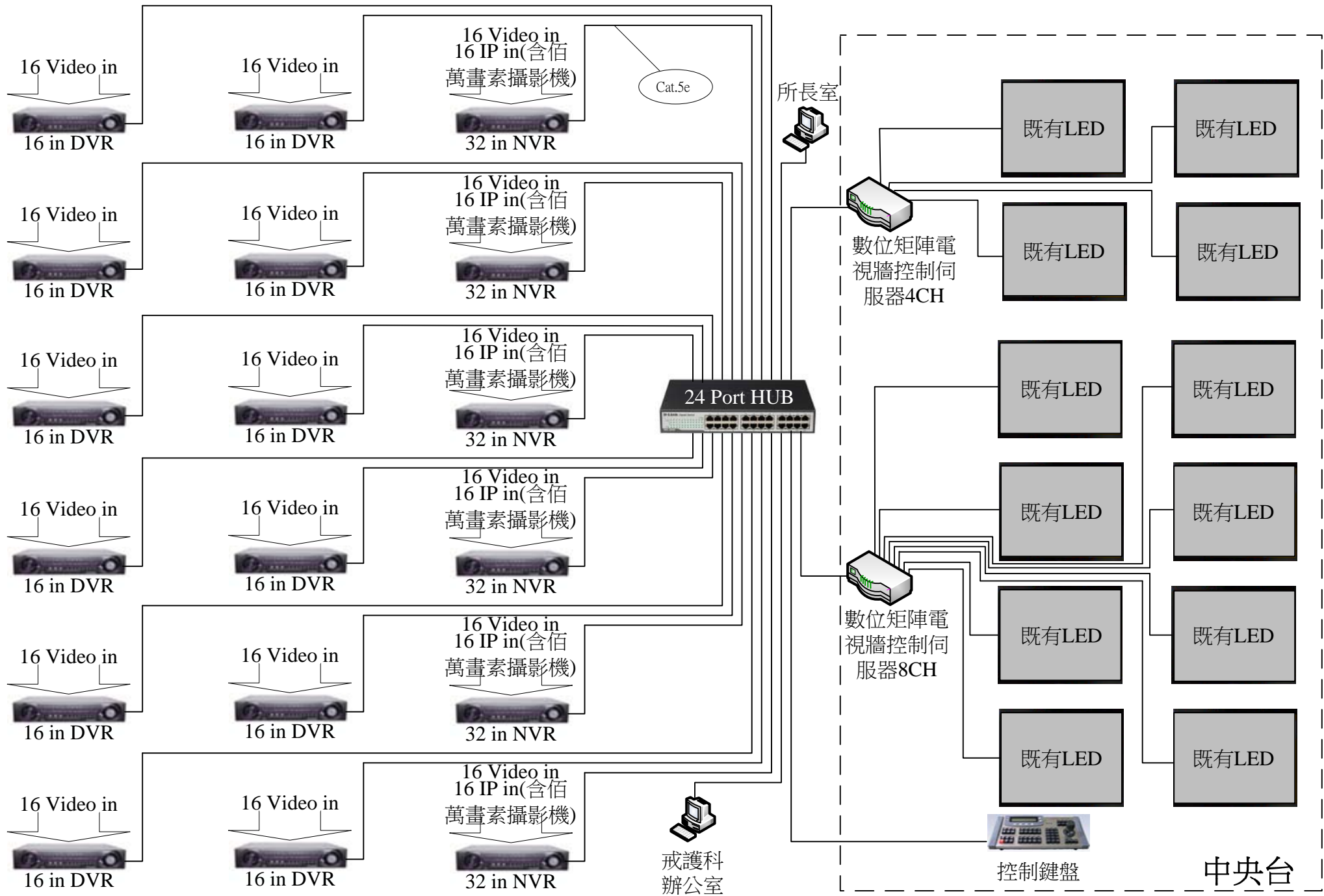
矯正署高雄戒治所監視錄影主機系統示意圖
